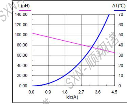
SMMS1360-101M
