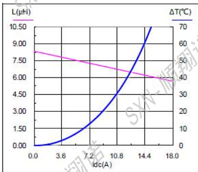
SMMS1360-8R2M
