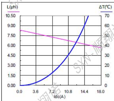
SMMS1360-8R2M
