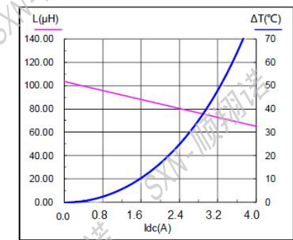
SMMS1040-101M
