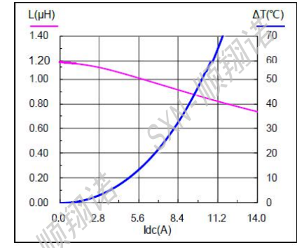
SMMS0530-1R2M
