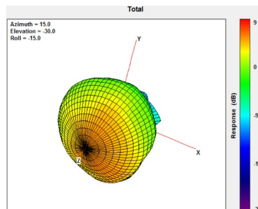
2170MHz
