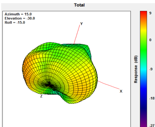
2690MHz
