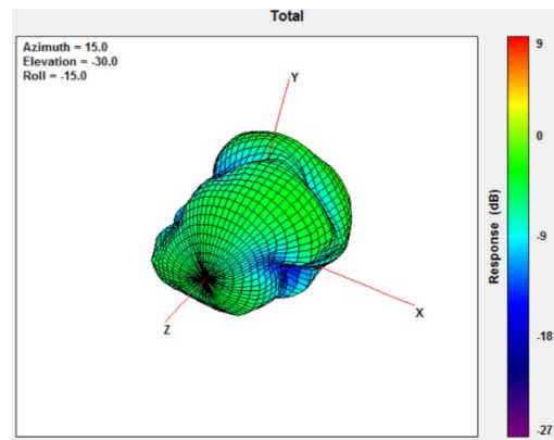
960MHz
