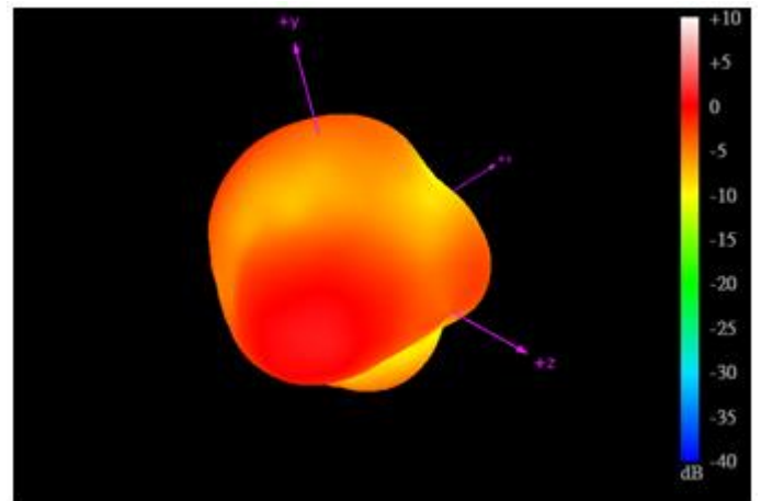
1602MHz
