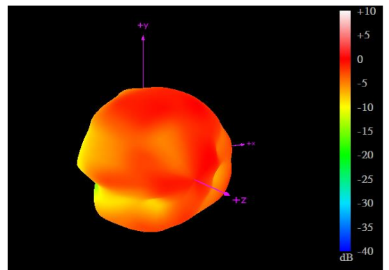
3500MHz
