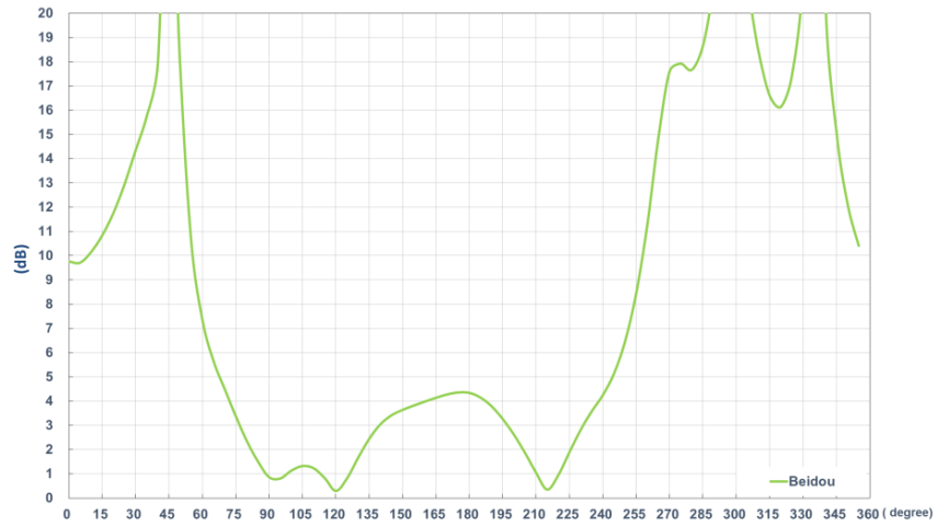
1561MHz
