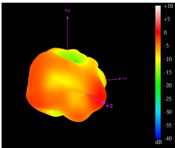
704MHz
