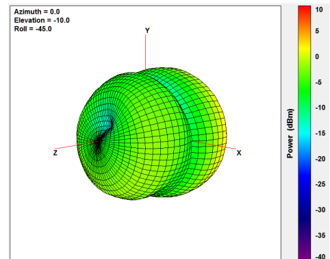
1990MHz
