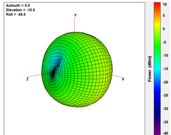
960MHz
