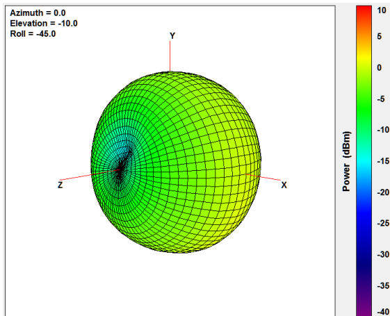
894MHz
