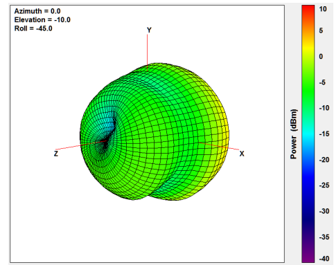
1805MHz
