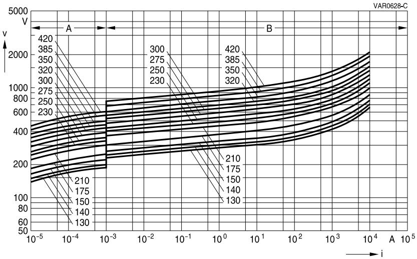
SIOV-ETFV20 ... E2
