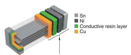
树脂电极品
