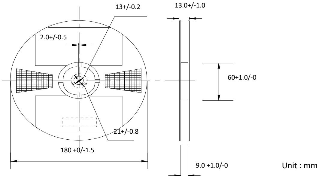
Reel Dimensions
