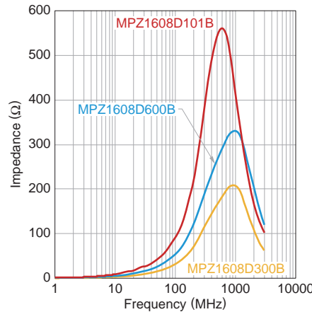
MPZ1608D 系列
