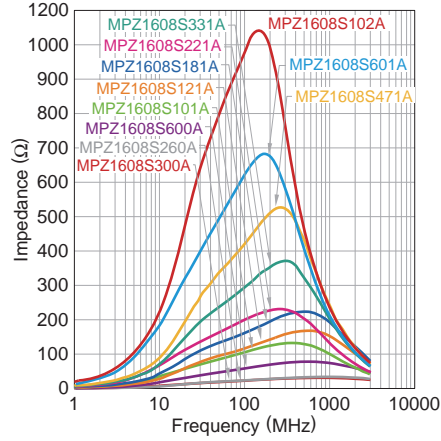
MPZ1608S 系列
