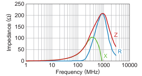
MPZ1608D300BTA00
