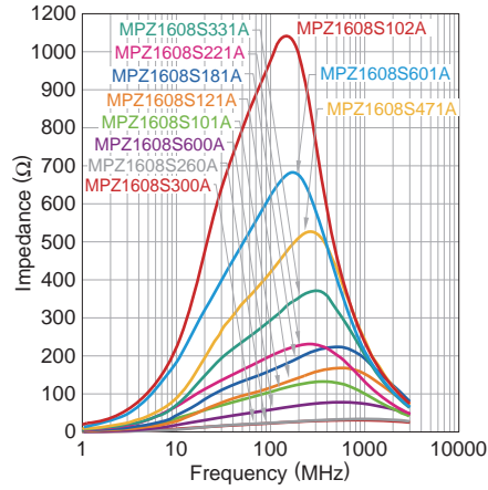
MPZ1608S 系列
