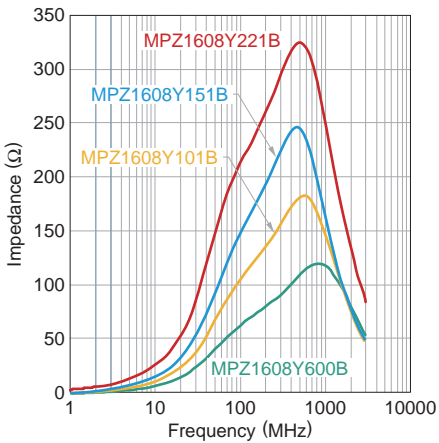
MPZ1608Y 系列
