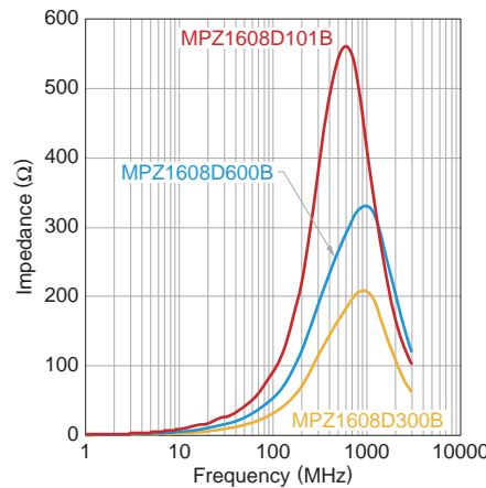
MPZ1608D 系列
