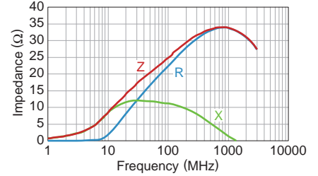
MPZ1608S121ATAH0
