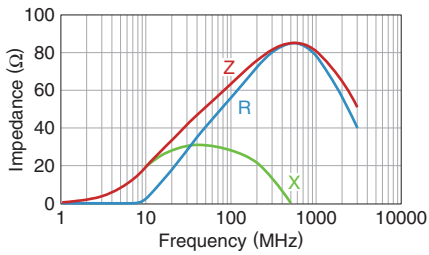
MPZ1608S181ATDH5
