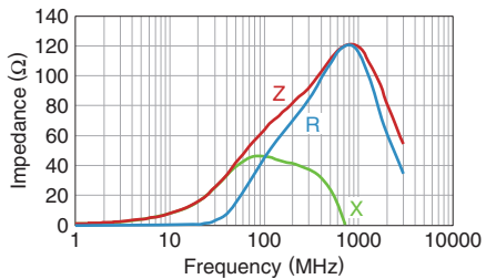
MPZ1608Y600BTD25
