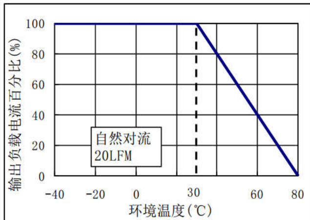
温度降额曲线图
