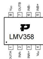
LMV358 (SOP8)
