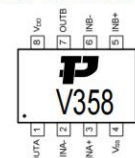
LMV358MMX-P (MSOP8)
