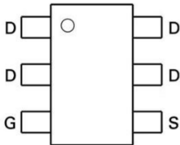
SOT23-6
