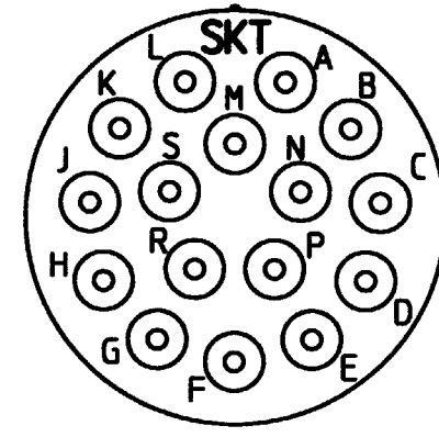
GROMMET SOCKET SIDE
