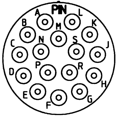
GROMMET PIN SIDE
