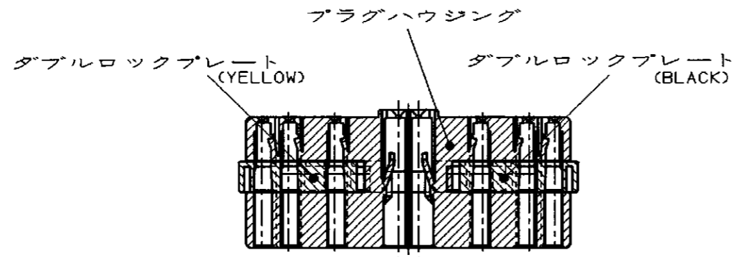
断面 A-A
