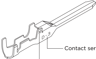
Tab contact
