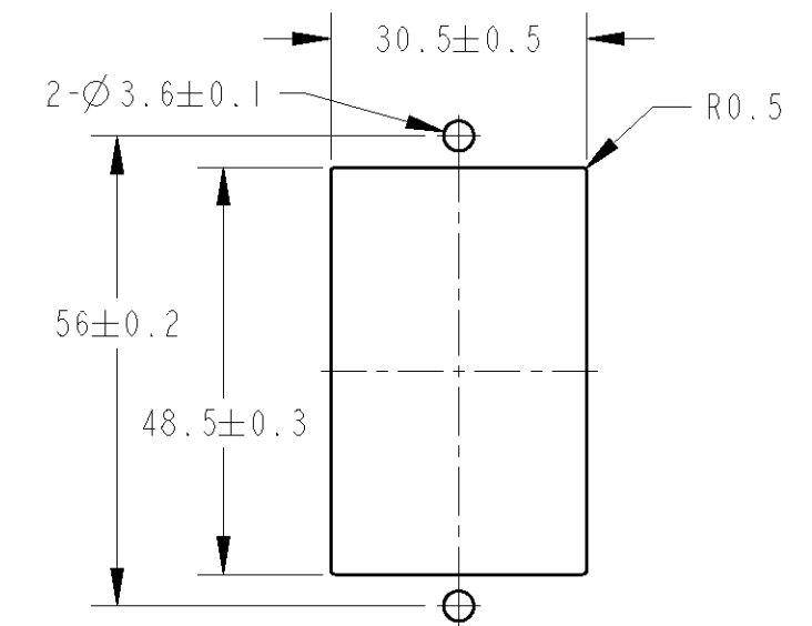
パネル加工推奨寸法図 RECOMMEND PANEL LAYOUT SCALE:1:1
