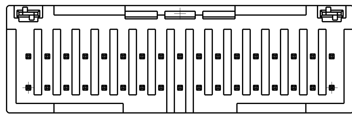
34POS(X-KEY):1-1827872-7
