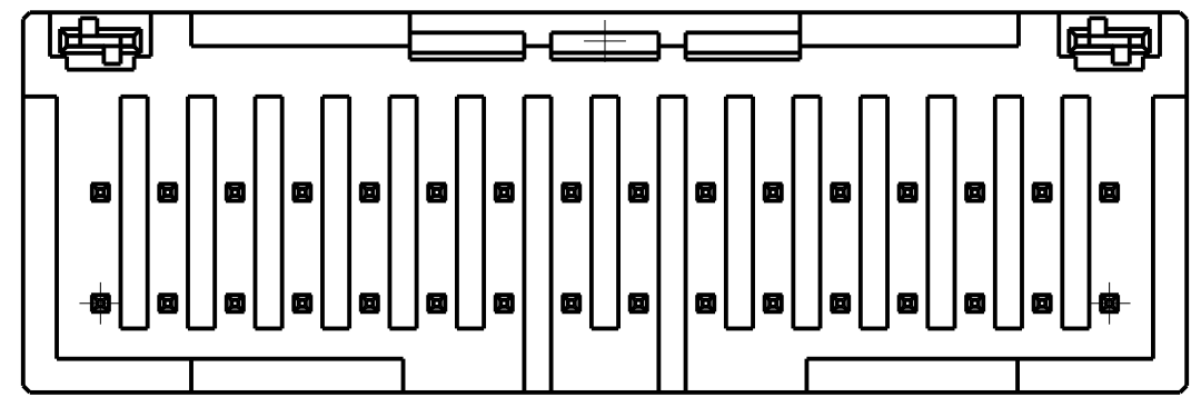
32POS(X-KEY):1-1827872-6
