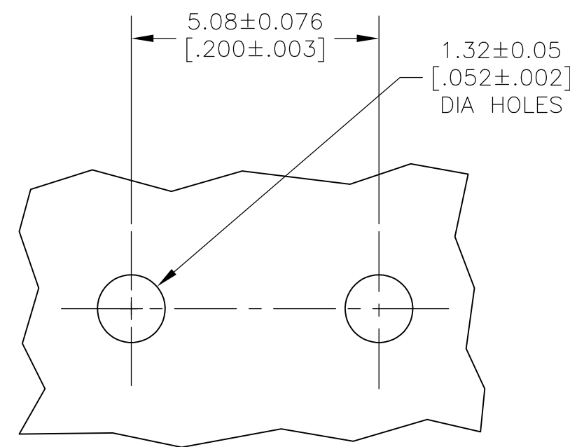
P.C.BOARD HOLES
