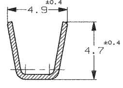
SEZIONE B-B (SECTION B-B)
