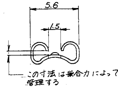
矢視 A-A
