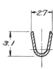
断面 B-B
