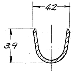
断面 C-C
