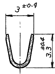
断面 A-A
