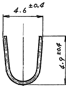
断面 B-B
