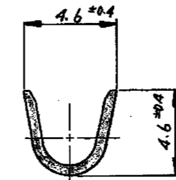
断面 'B-B' (SECTION "B-B")
