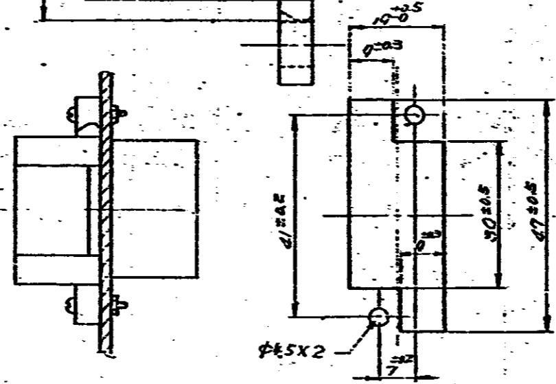
パネル打抜き寸法と取付位置 PANEL CUTTING DIMENSIONS
