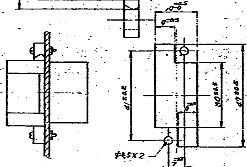
パネル打抜き寸法及び取付寸法 PANEL CUTTING DIMENSIONS
