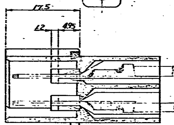
断面 A-A
