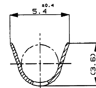
SECT. 断面 C-C
