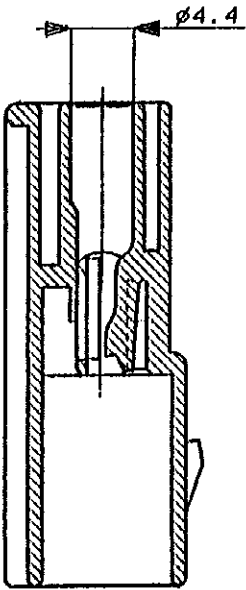
SECTION A-A 断面 A-A
