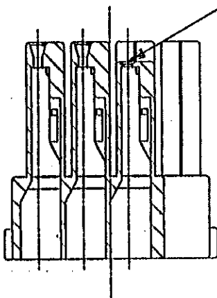
断面 A-A SECT.
