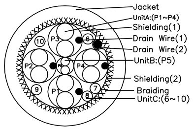
A-A VIEW
