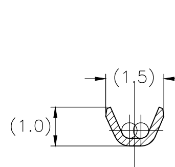
断面 B-B SECT.
