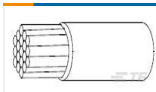
TE Part #216441-000 22759/33-24-0
