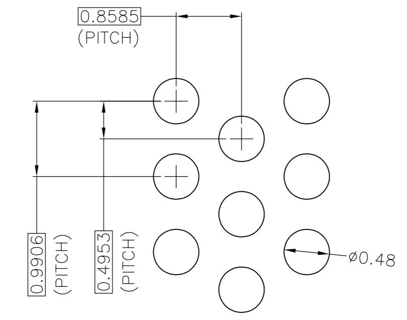
DETAIL M(20:1)
