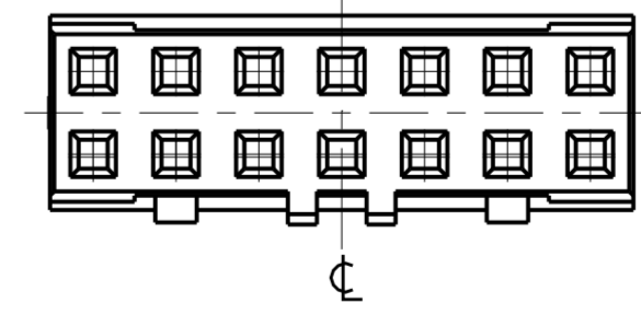
SCALE 5:1
