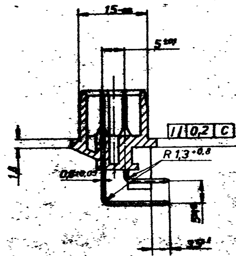
Schnitt A-B
