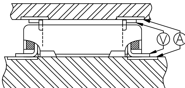
Fig.4 ローレベル総合抵抗測定方法 Method of Termination Resistance Measuring
