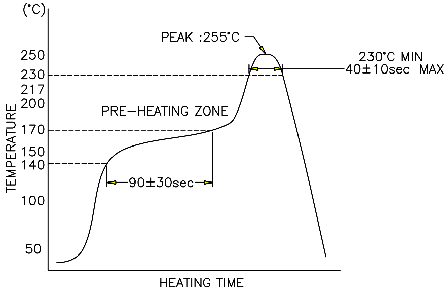
Fig.6 リフロー耐熱性の温度プロファイル Temperature Profile of Reflow Resistance solder heat
