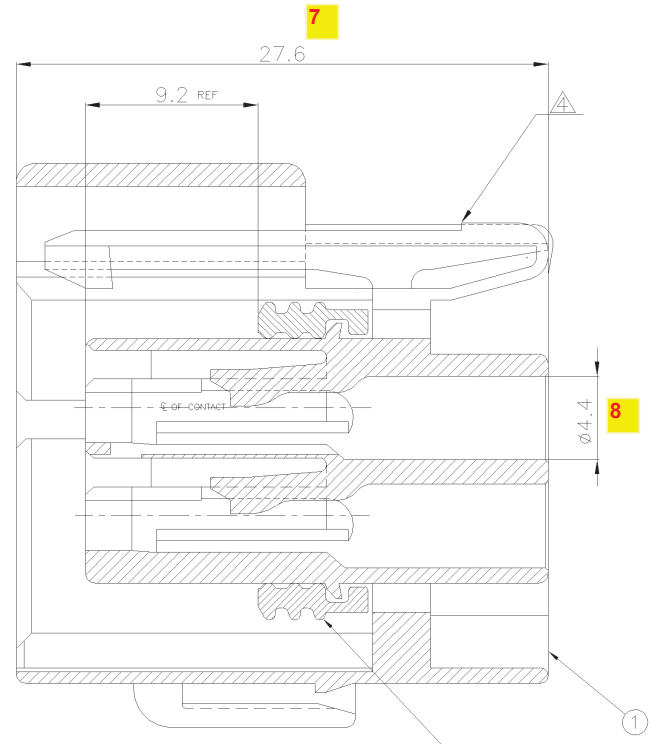
SECT A-A
