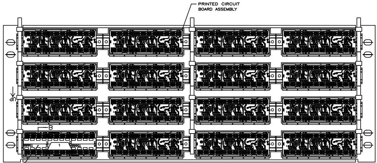
VIEW A-A
