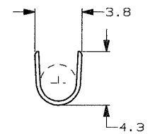
SEZIONE B-B (SECTION B-B)
