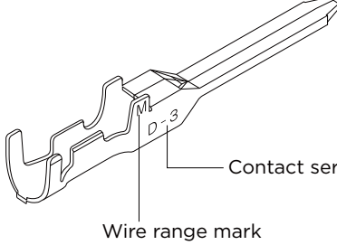
Tab contact
