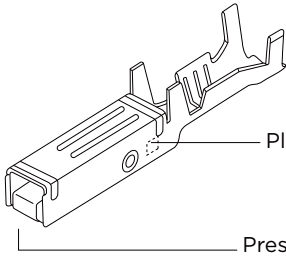
Receptacle Contact
