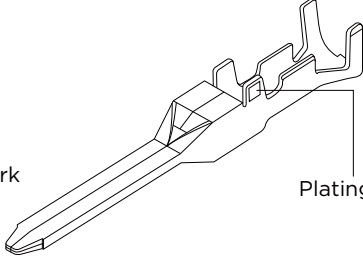
Tab contact
