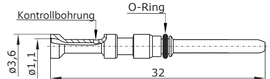
Hauptabmessungen Kontaktstift
