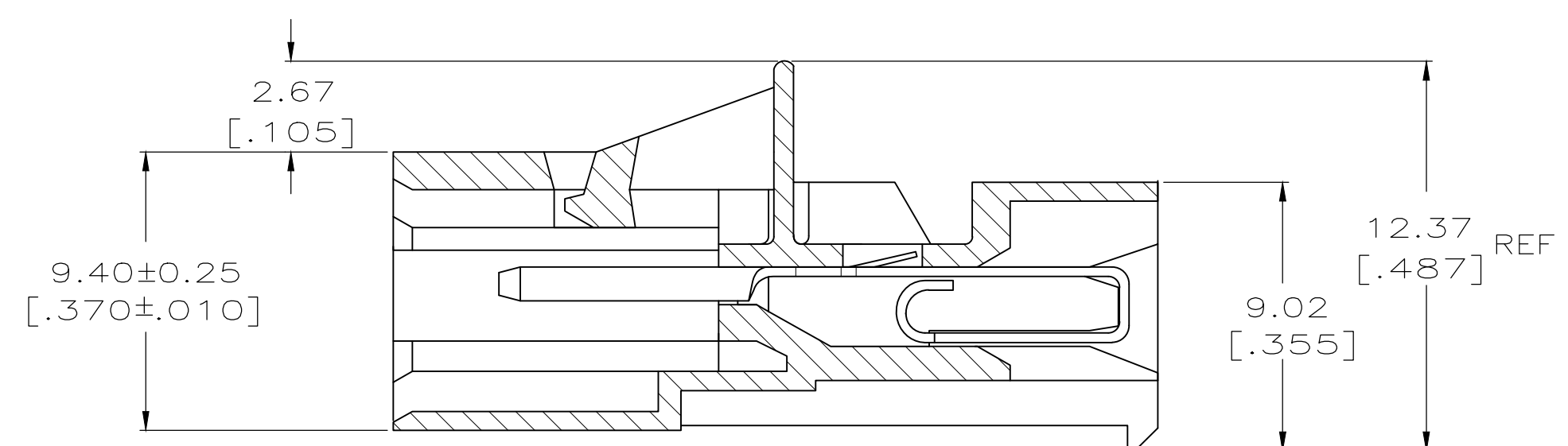
SECTION A-A
