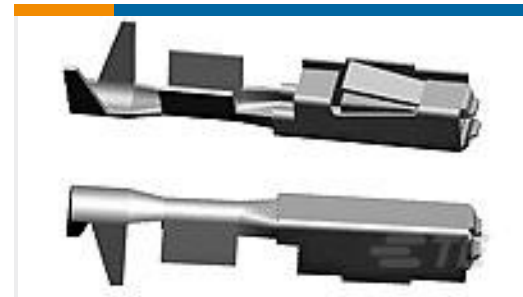
TE Part # 5-962885-5 MQS0,63 Au rec LL EDS 0,2-0,35
