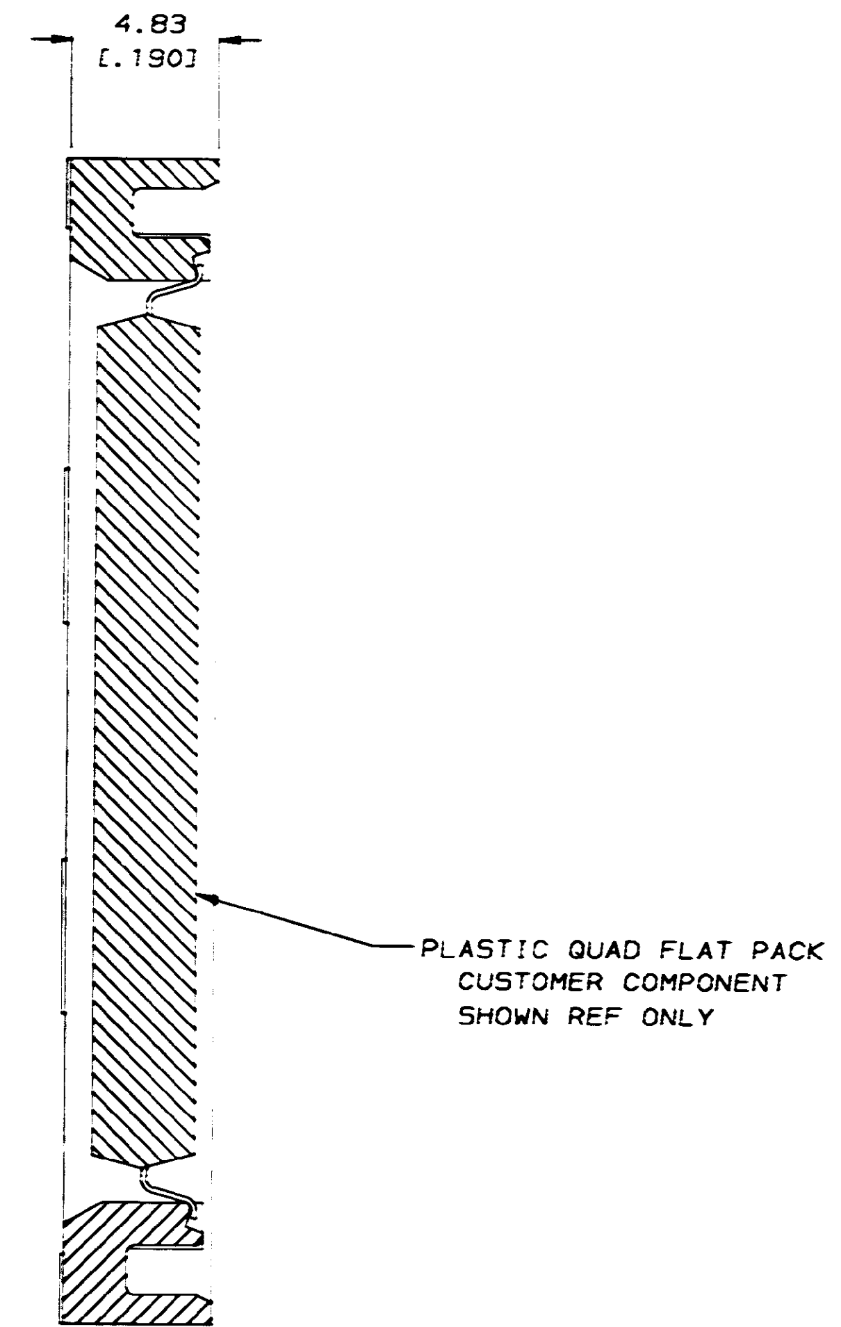
SECTION A-A
