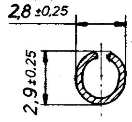
Schnitt A-A
