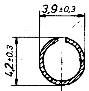
Schnitt B-B
